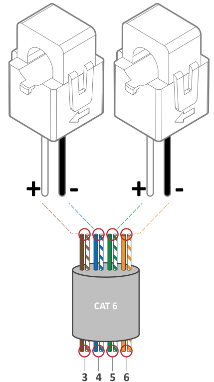
Extensión de sensores CT con cable CAT 6
